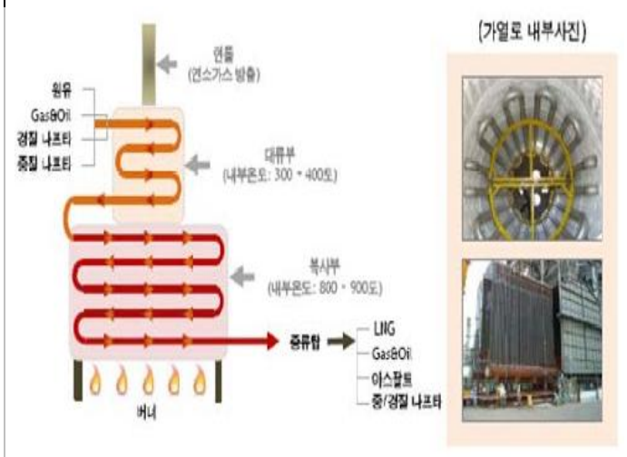
그림 2. 가열로의 구조
